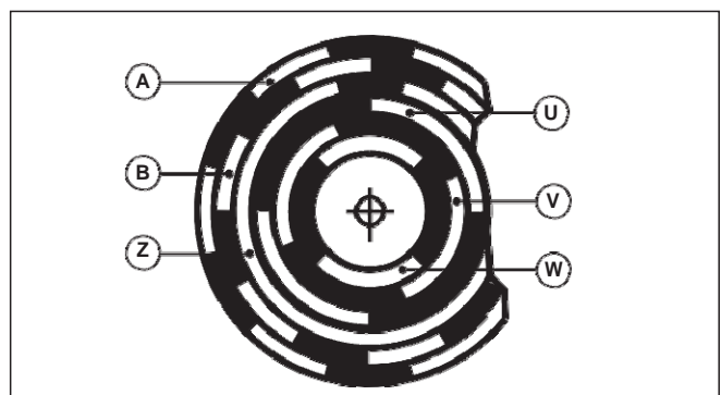
Representación gráfica de las señales incrementales A,B, y Z con fases de conmutación U,V y W.
