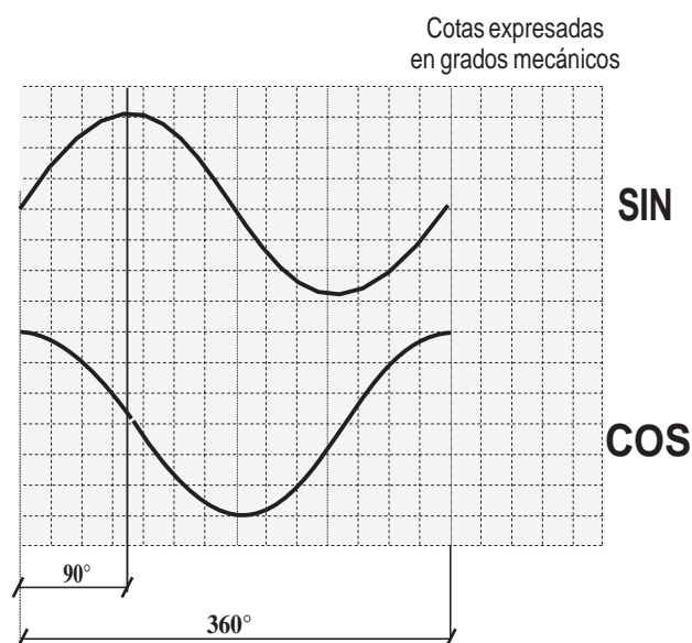
Representación gráfica de las señales de conmutación sin y cos
