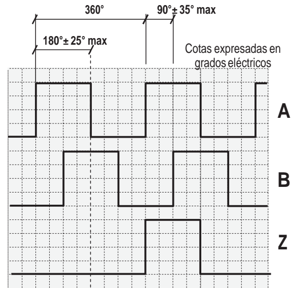
Representación gráfica de las señales incrementales A,B, y Z.
