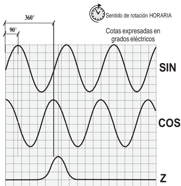
Representación gráfica de las señales sinusoidales sin, cos y Z.
